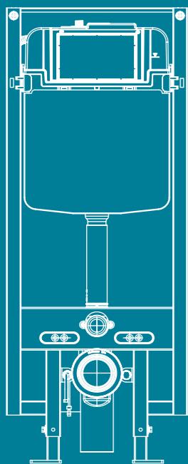
Комплект: Застенный модуль с унитазом-биде и панелью смыва TECEspring R
